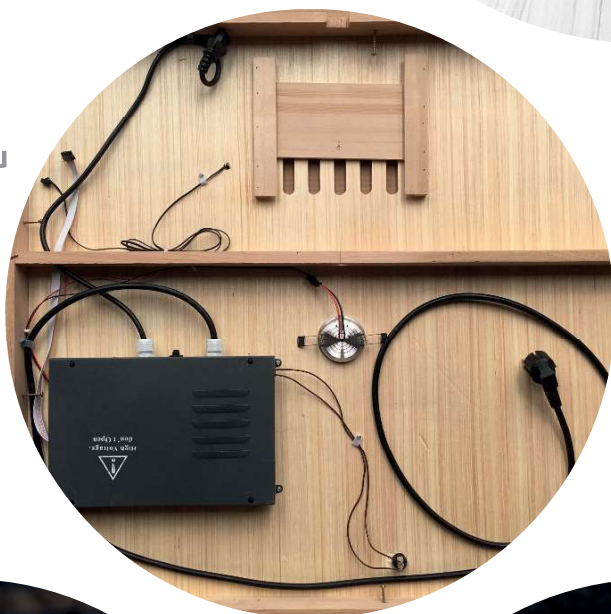
Ukážka pretiahnutie káblov
